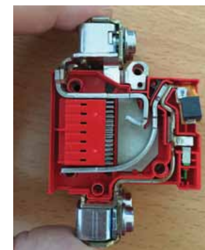
Detail uspořádání jiskřiště v DEHNshield
